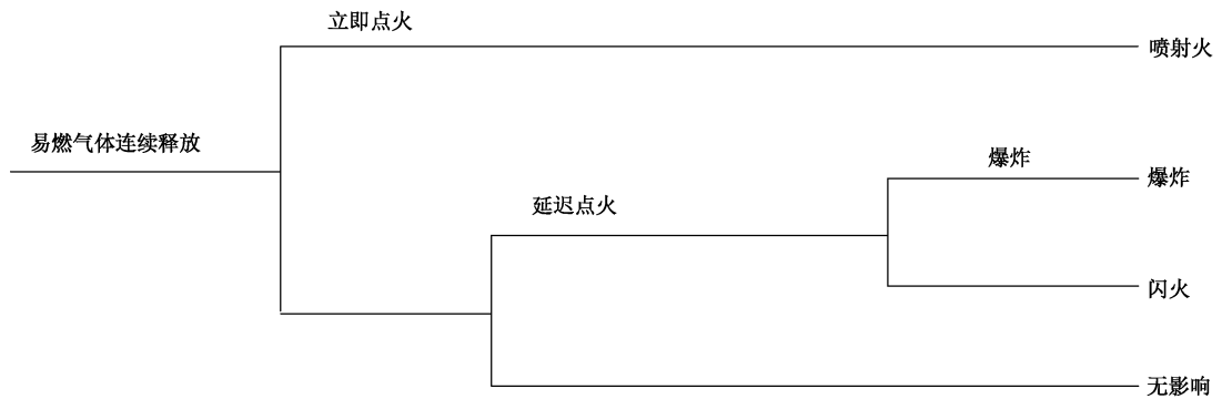
图 F.2 易燃气体连续释放事件树
