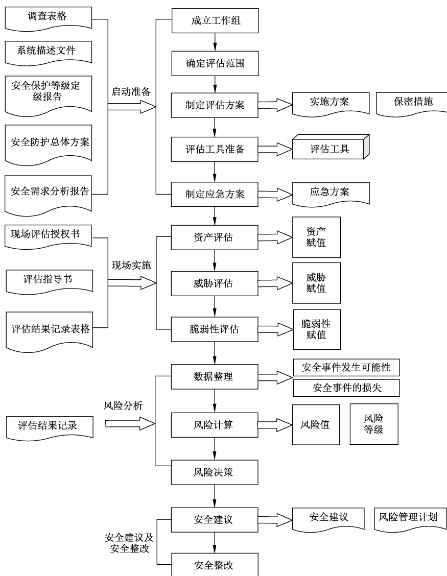
图1 电力监控系统网络安全评估实施流程
