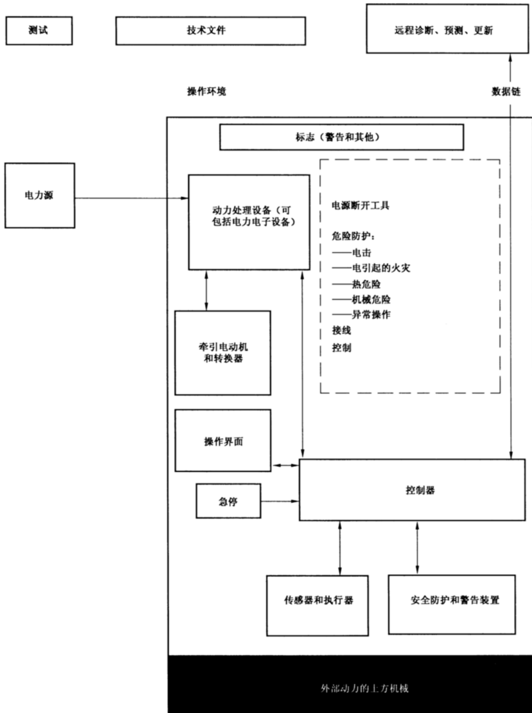
图 1 典型机器框架图
