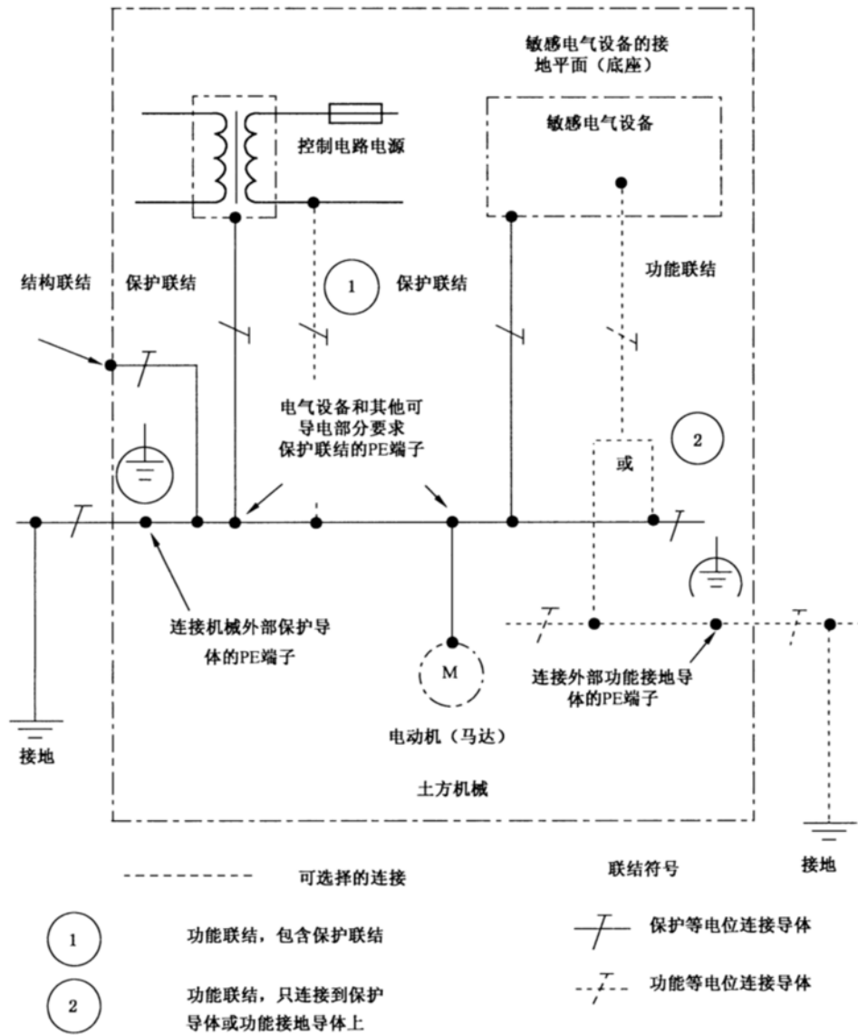
图2 机械电气设备等电位联结示例
