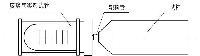
图 1 以体积为计量单位的杀虫气雾剂净含量测定装置
