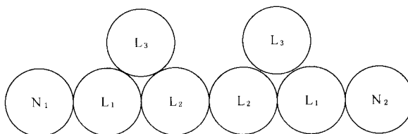
图 H.52.3 三角形方式敷设排列的 6 根并联单芯电缆(见 523.7)
