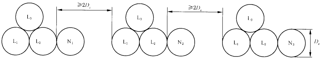
图 H.52.5 上下层方式敷设排列的 9 根并联单芯电缆(见 523.7)
