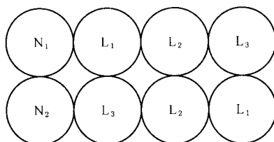
图 H.52.1 平排方式排列的 6 根并联单芯电缆(见 523.7)
