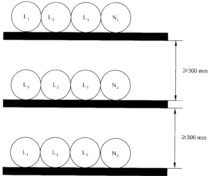
图 H.52.4 平排方式敷设排列的 9 根并联单芯电缆(见 523.7)
