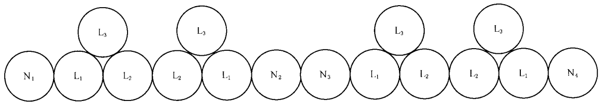
图 H.52.8 上下层方式敷设排列的 12 根并联单芯电缆(见 523.7)
