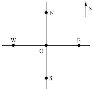
图 A.1 地电场测量电极布极示意图
