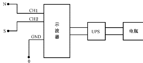
图 A.3 测量设备连接框图
