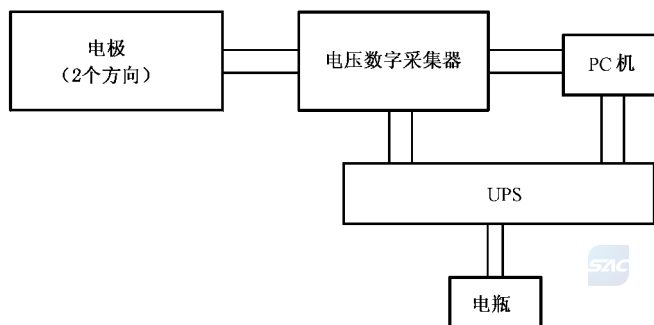
图 A.2 地电场测量系统连接框图
