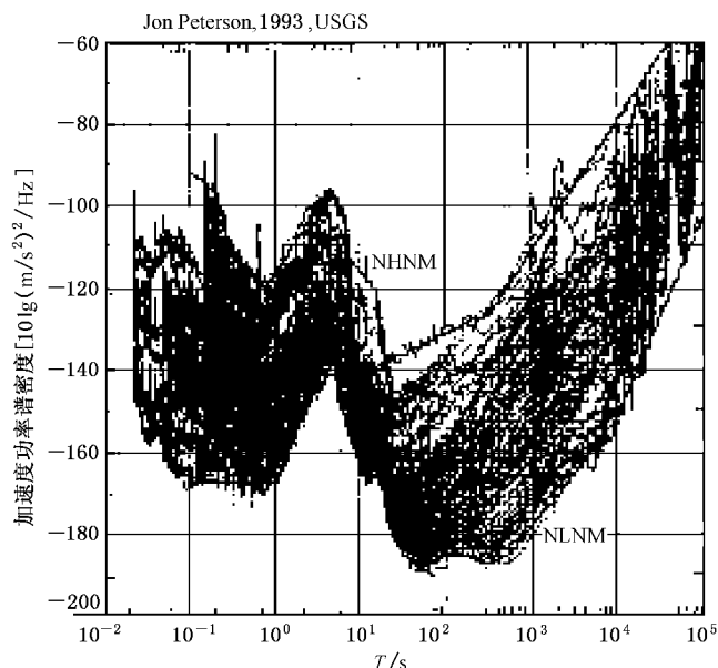
图 A.1 地球噪声模型(Peterson, 1993)
