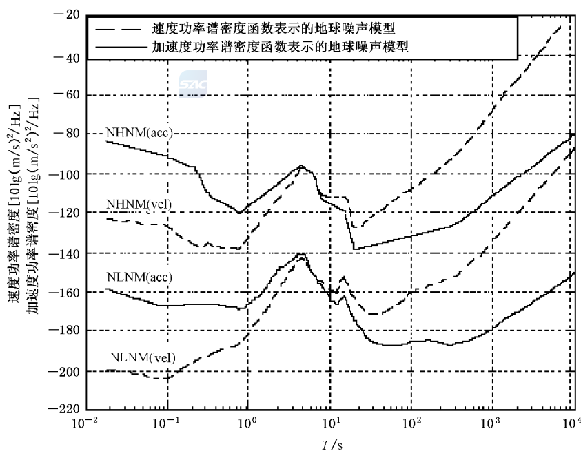
图 B.1 地球高噪声模型(NHNM)和低噪声模型(NLNM)
