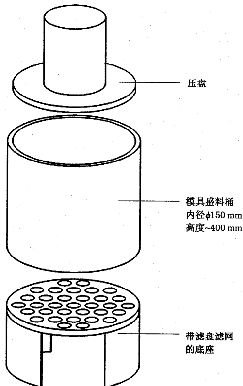
图 A.1 模具示意图
