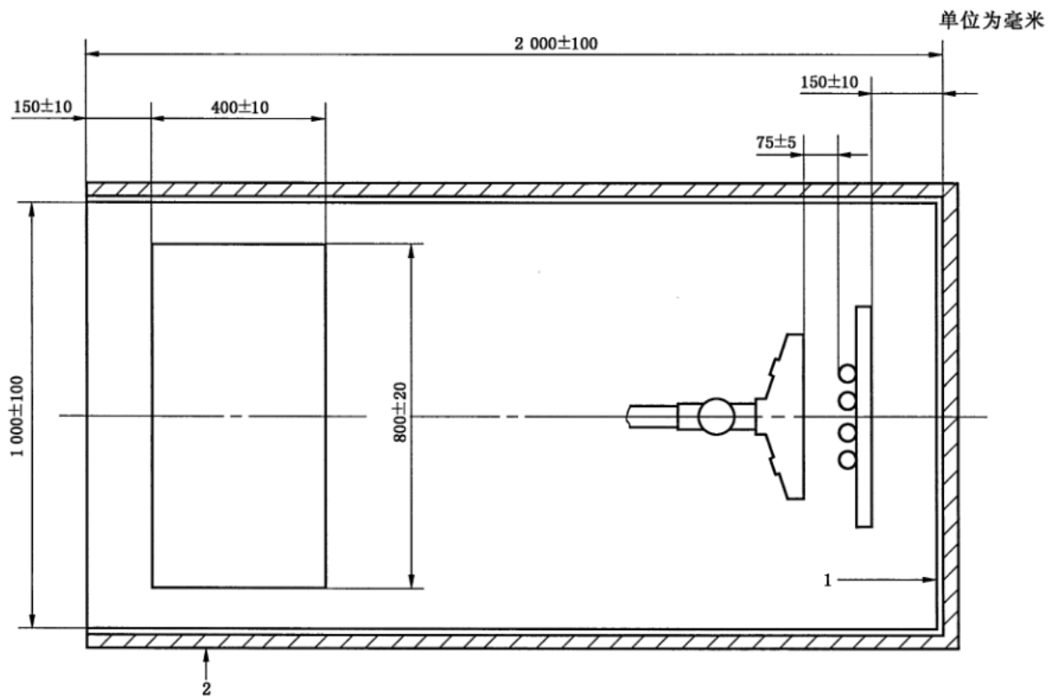
图 1 试验箱（续）
