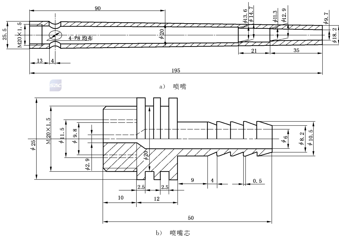
图 1 喷嘴
