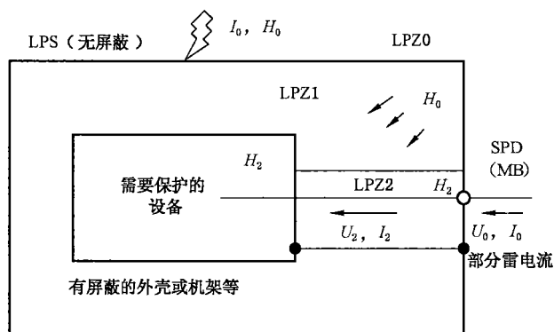
注：设备得到防线路导入电涌的保护， U_2 小于 U_0 和 I_2 小于 I_0 ，以及 H_2 小于 H_0 。防辐射磁场的保护。
