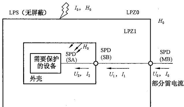
注：设备得到防线路导入电涌的保护， U_2 远小于 U_0 和 I_2 远小于 I_0 ，但不需防 H_0 。辐射磁场的保护。
