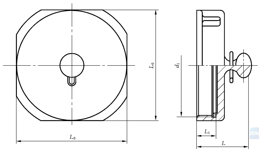
图 2 KA 型阀盖
