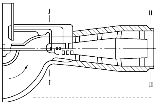
图 2 轴流式通风机测压断面位置图
