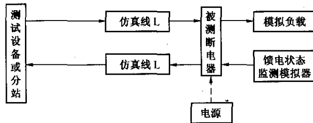
图 1 试验线路
