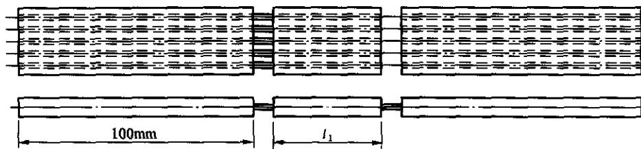
图 B.2 钢丝绳黏合强度试件
