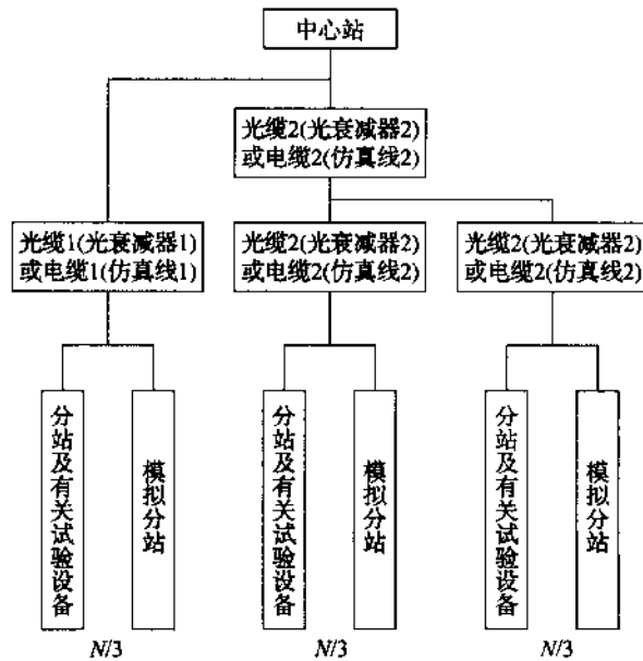
图 1 树形系统设备连接
