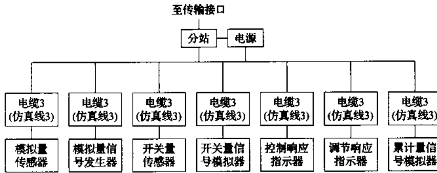
图 4 分站设备连接
