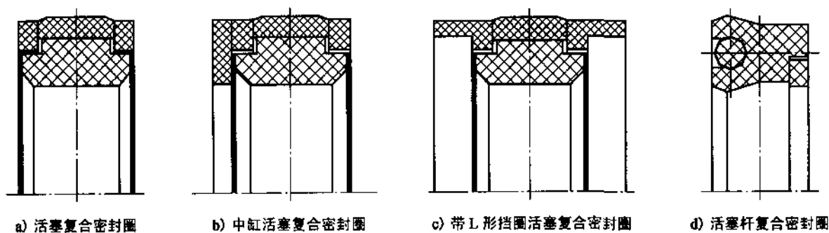
图 4 复合密封圈结构型式
