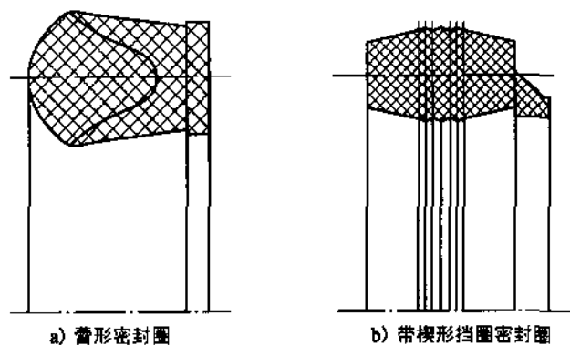
图 3 活塞杆单体动密封圈和挡圈结构型式
