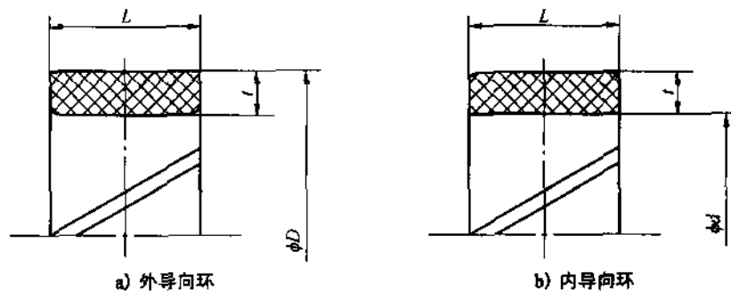
图6 导向环结构型式
