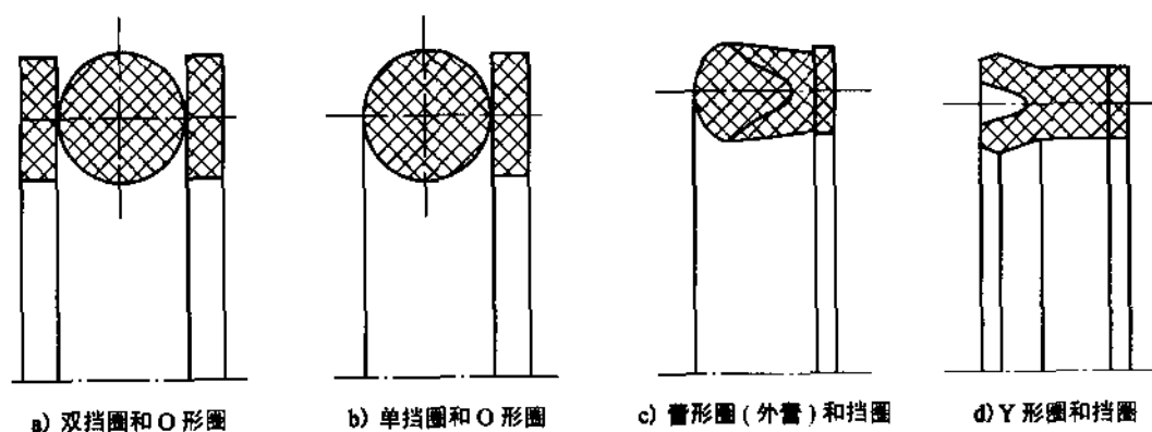
图1 单体静密封圈和挡圈的结构型式
