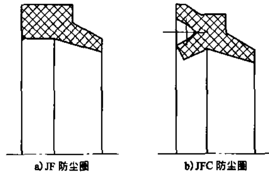
图5 防尘圈结构型式
